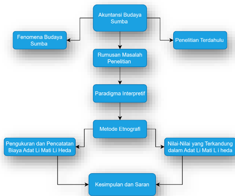
Gambar 1. Kerangka Pemikiran
